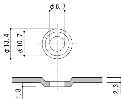
エンボス加工部詳細図 S=1/1
